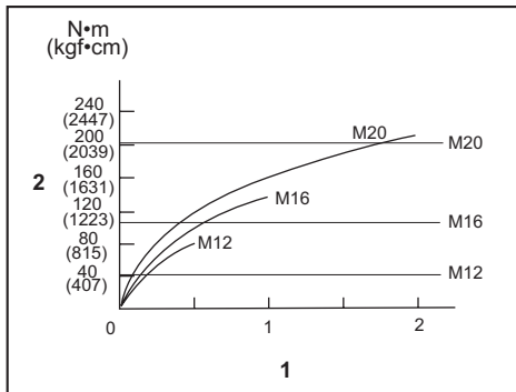
1. Durée de serrage (en secondes) 2. Couple de serrage
