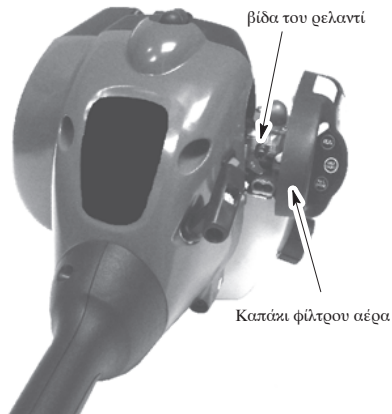
βίδα του ρελαντί
