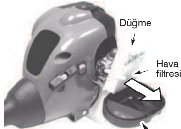
Hava filtresi kapağı
