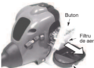
Capacul filtrului de aer
