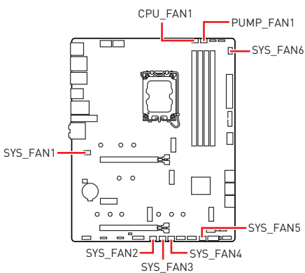
风扇接口规格
