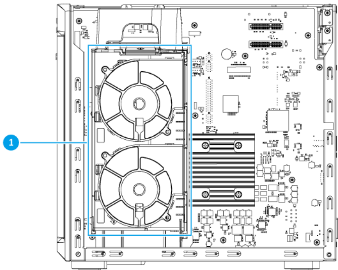
Modulo ventola collegato
