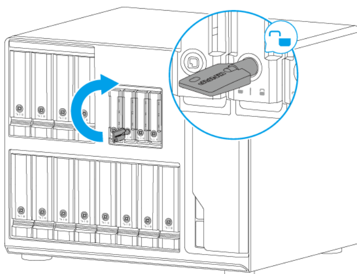
TVS-h1688X
