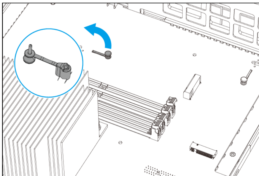
M.2 2280
