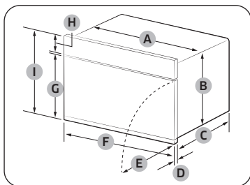
Gerät (mm)
