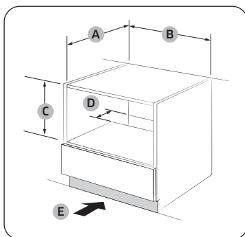
Unterbauschranks (mm)
