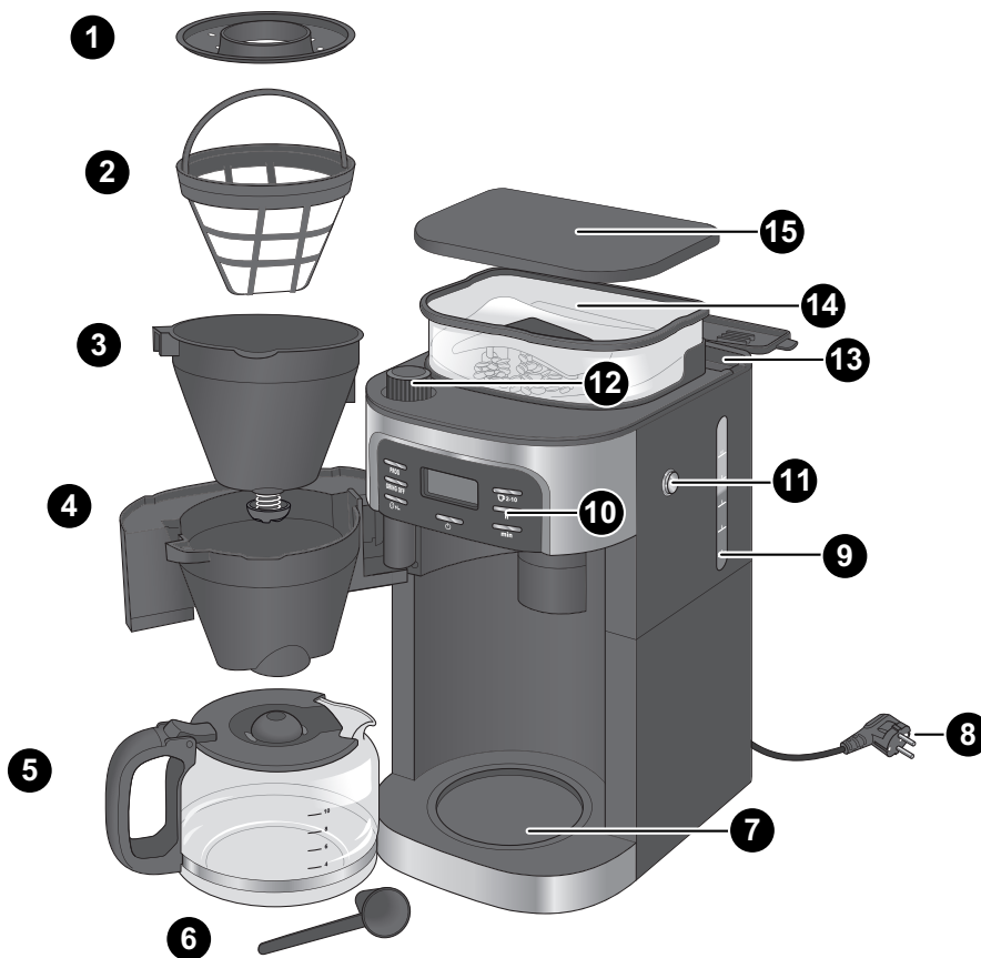
Fig. 1: Apparatets dele
