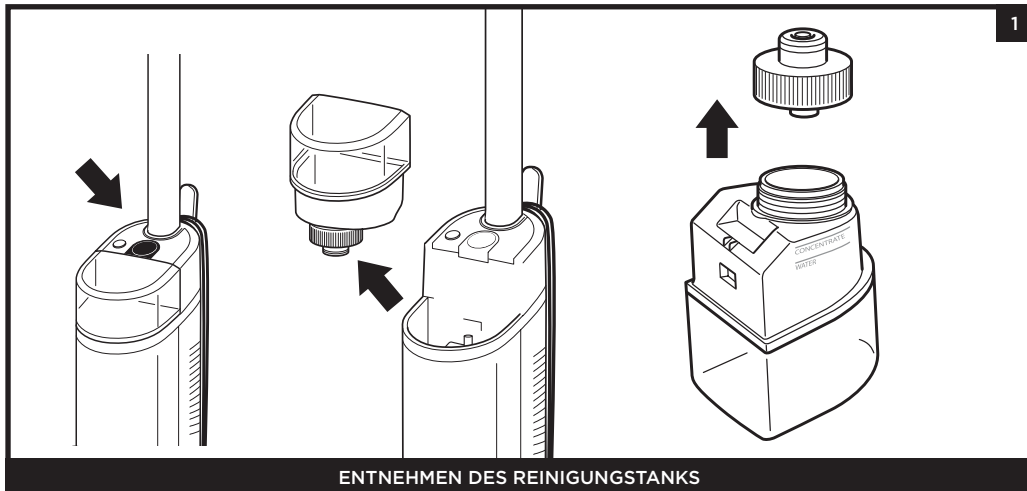
ENTNEHMEN DES REINIGUNGSTANKS
