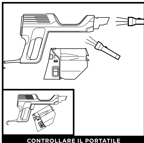
CONTROLLARE IL PORTATILE
