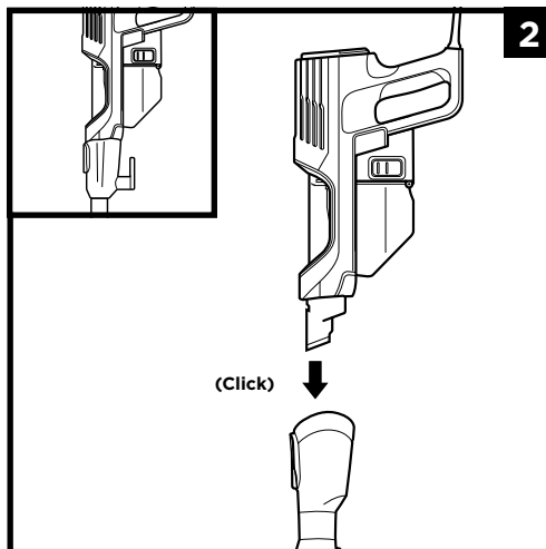
2. Sätt i handenheten i röret.
