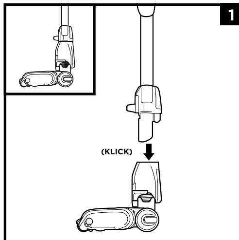
1. Stecken Sie das Rohr in die Bodendüse .
