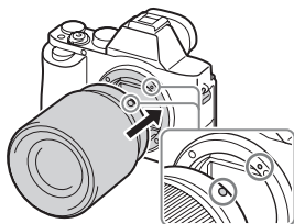
Weißer Ausrichtmarkierungen
