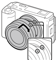
Monteringsmärken
