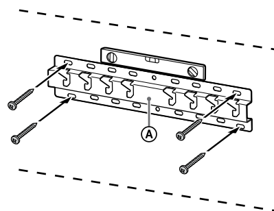
Ex.: Montering av bas (20) Ⓐ på plats "a"
