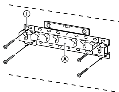
Ex.: Montering av bas (20) Ⓐ på plats "a"
