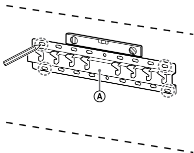
Ex.: Markering av plats "a" för montering i bas (20) Ⓐ
