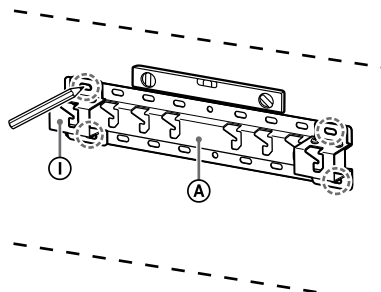
Es., marcatura nella posizione "a" per fissare la base (20) ③
