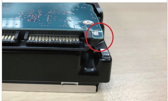
Bent PCB
