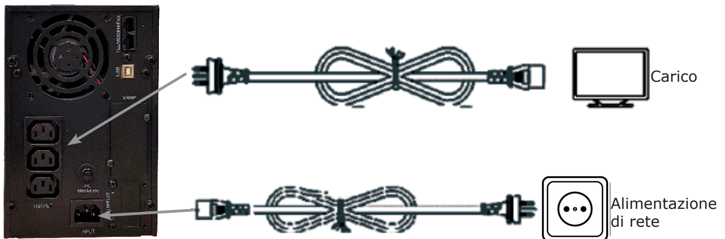
UPS Tower 1-2KVA Schema di collegamento ingresso/uscita
