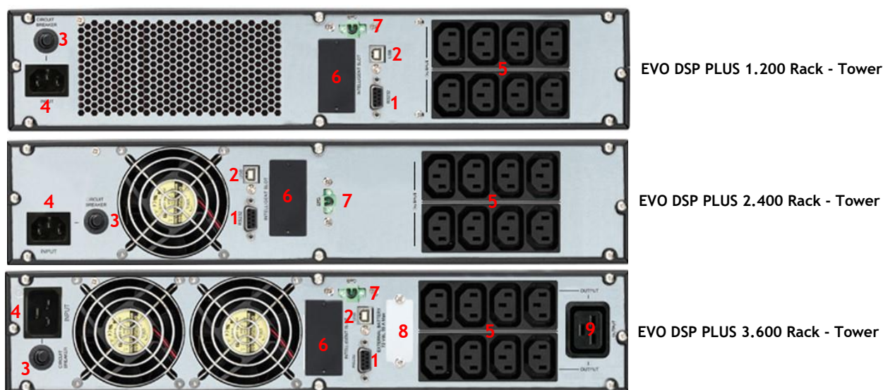
Figura 4 - Pannello Posteriore
