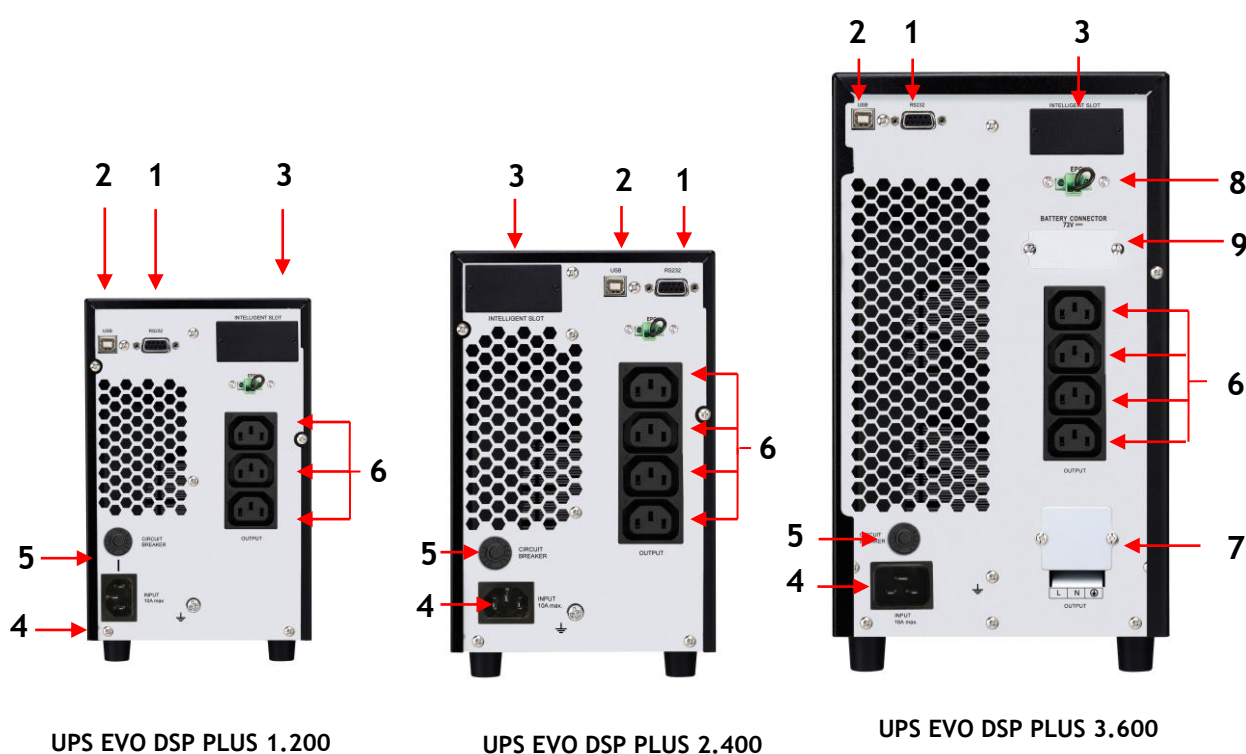
Figura 4 - Pannello Posteriore
