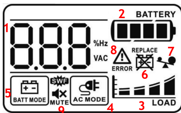
Figura 2 - Display LCD
