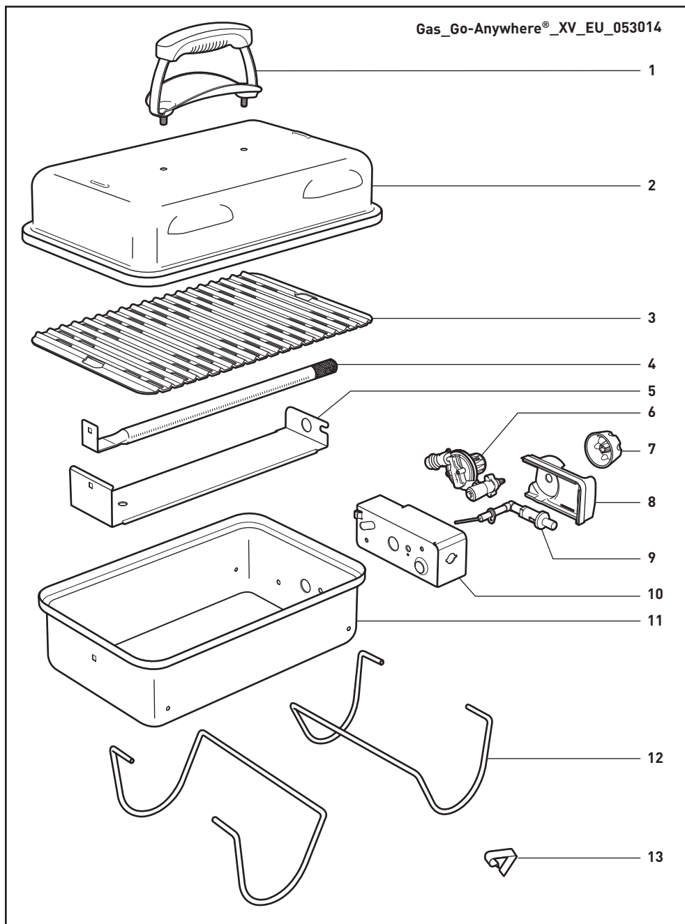
1. Maniglia
