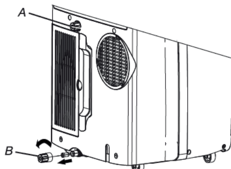
A. Bouchon de vidange secondaire
