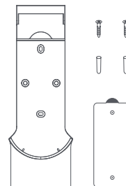
Крепление для зарядки и хранения "2 в 1" (в комплект входят 2 винта, 2 дюбеля и наклейка с монтажным шаблоном)
