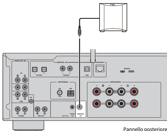
Pannello posteriore
